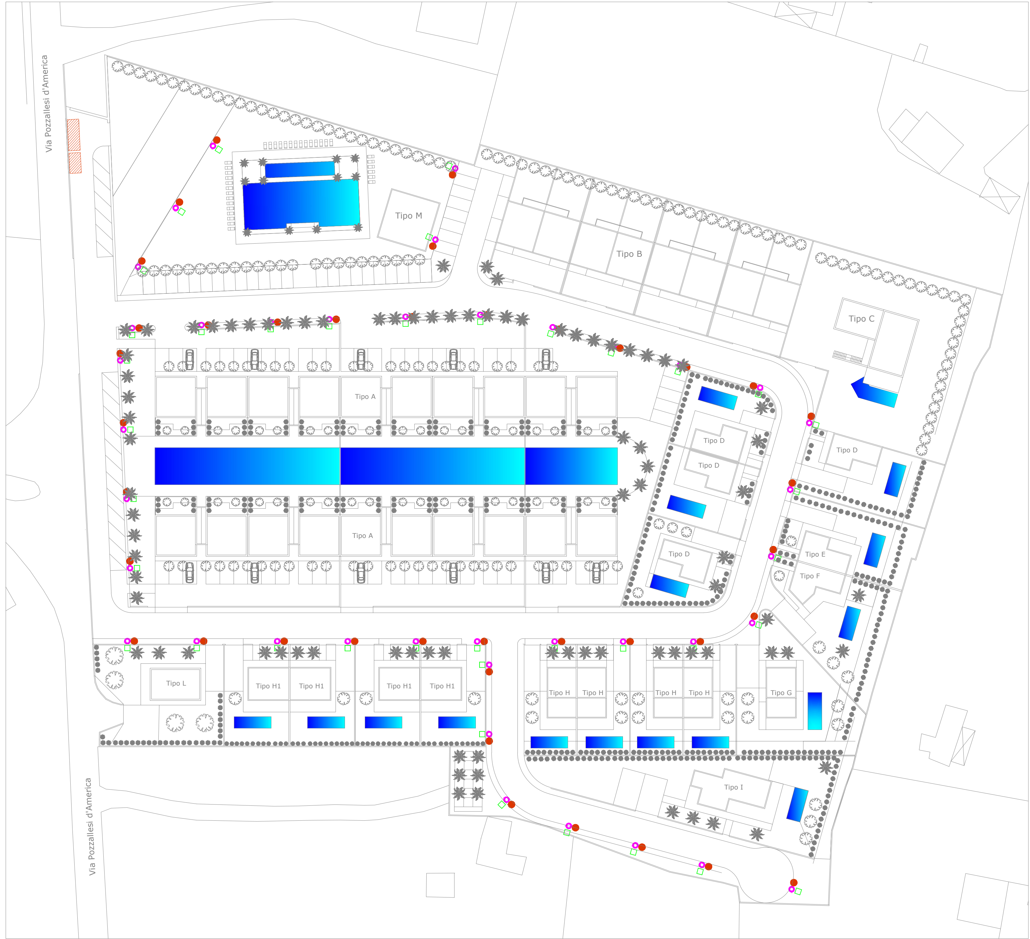
Planimetria Generale Corpi Illuminanti
